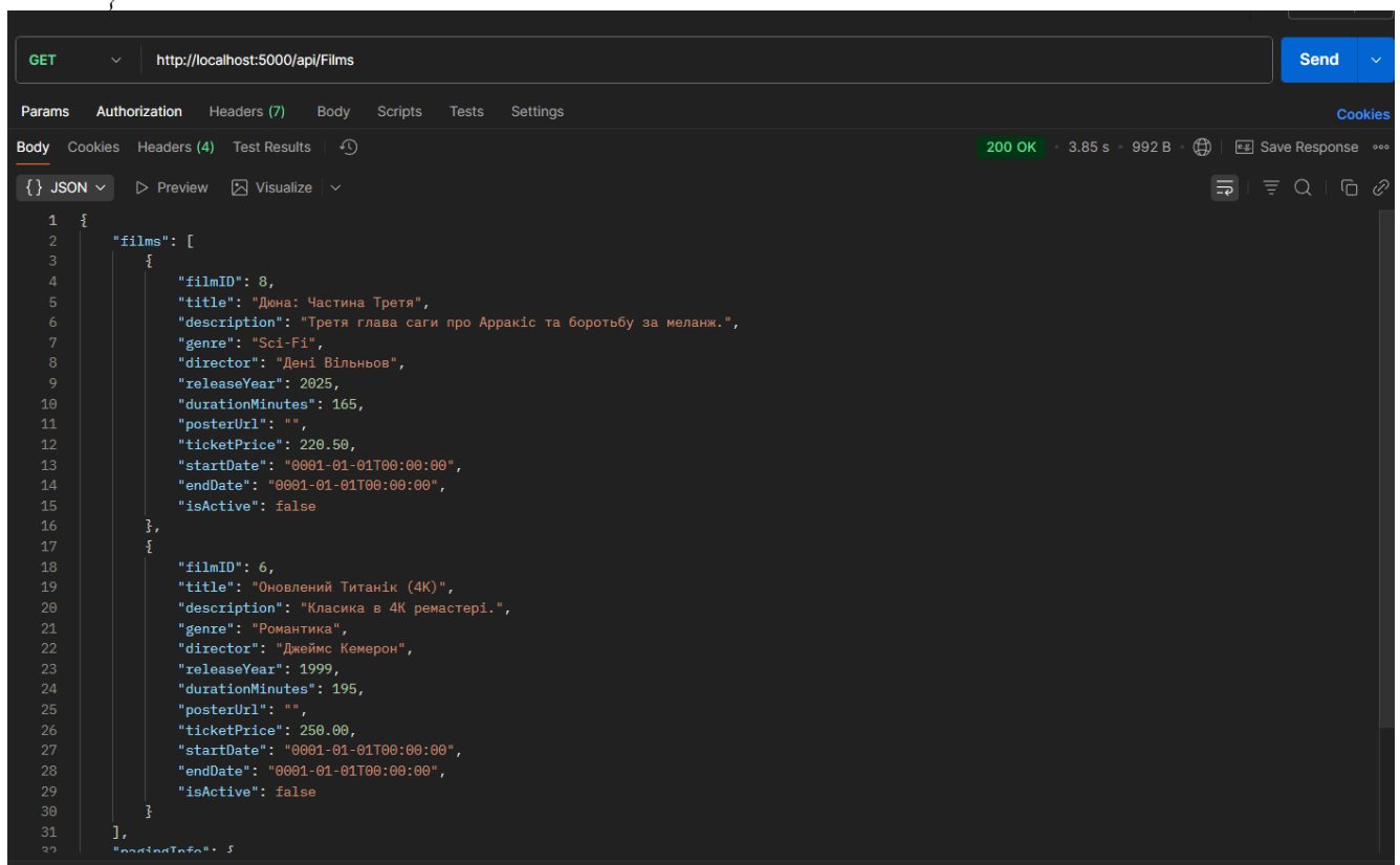
Рис. 5. Перегляд у postman
